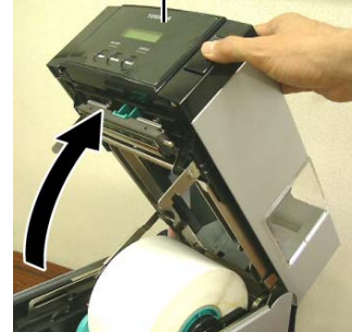
Gehäusedeckel
