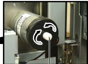
Messermotorschacht
